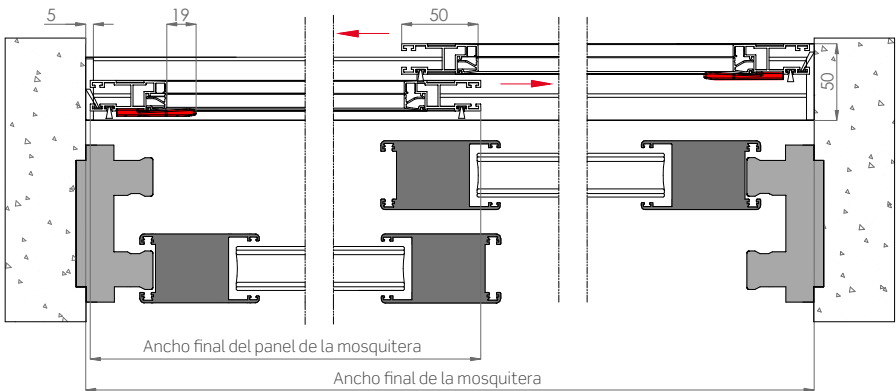
Sección horizontal
