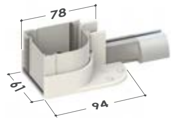
Cajón de 55 Cabezal inferior
