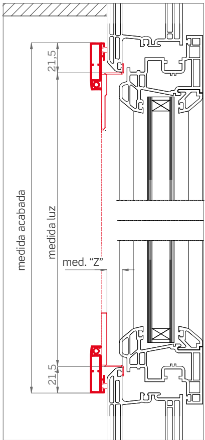
Sección vertical
