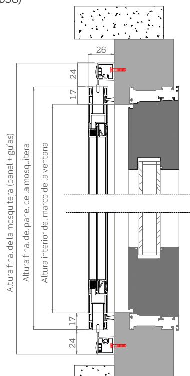
Sección vertical
