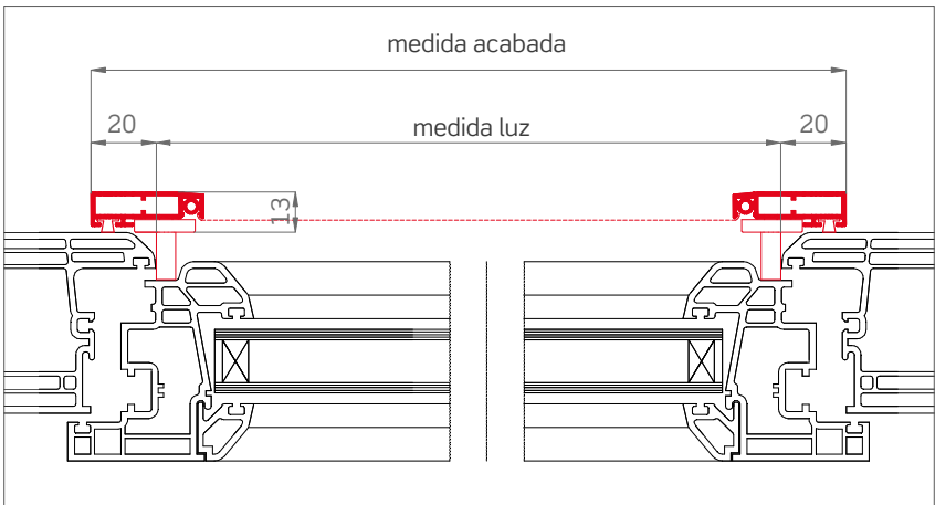
Sección horizontal
