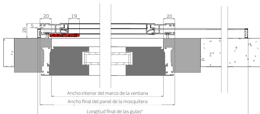
Sección horizontal
