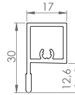
Guía superior (ZAP03G)
