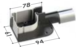
Cajón de 55 Cabezal inferior
