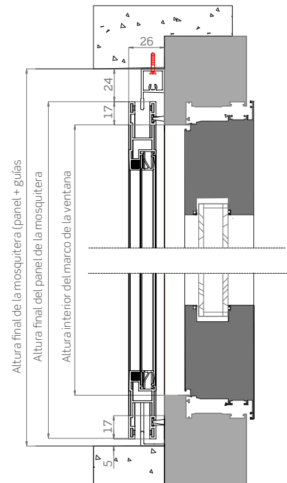
Sección vertical
