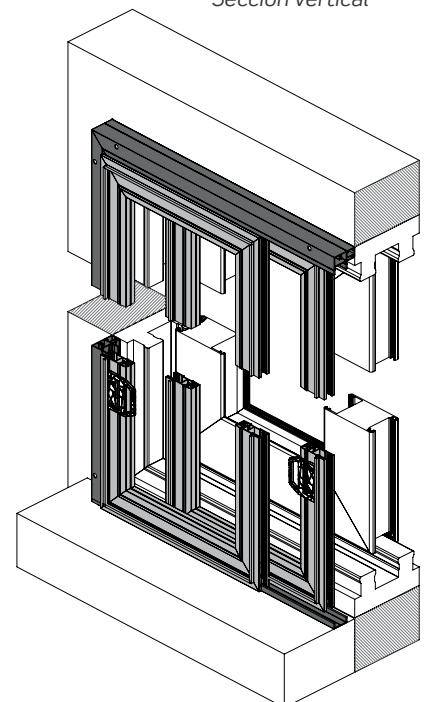
Sección vertical
