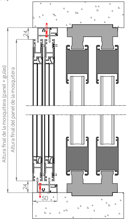
Sección vertical
