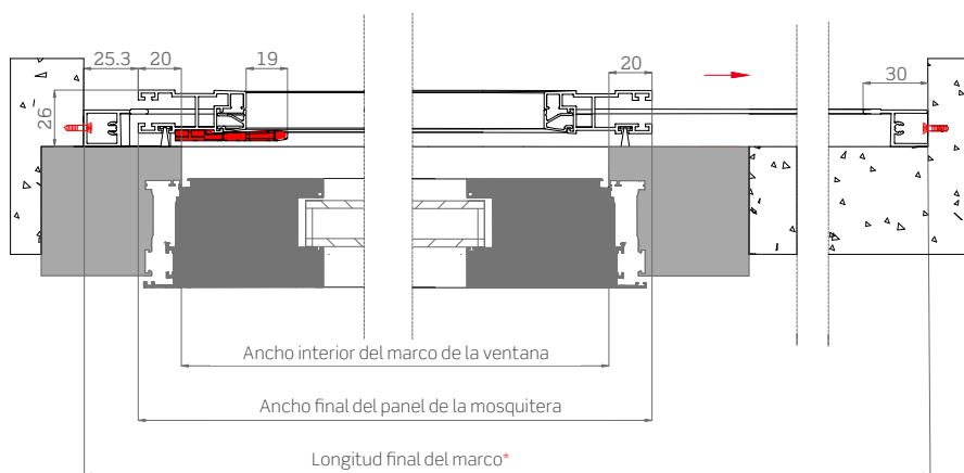
Sección horizontal
