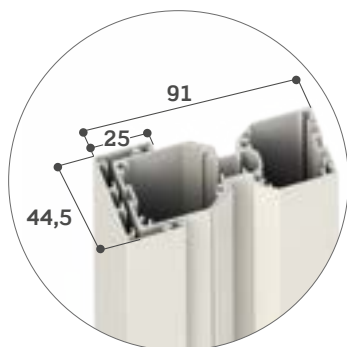
Recogida con perfil de cierre
