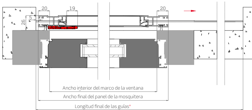
Sección horizontal
