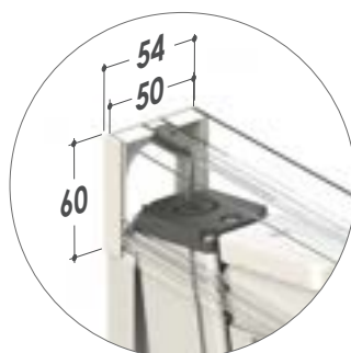
Conexión de bayoneta
