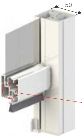
Barra con manija y perfil portacepillos telescópico (hasta 8 mm).
