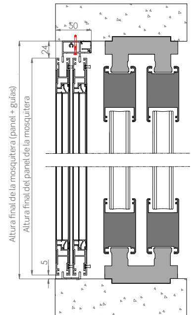
Sección vertical
