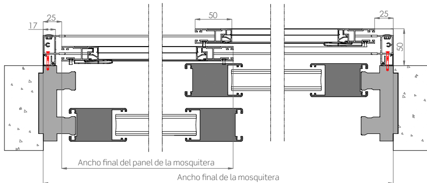
Sección horizontal
