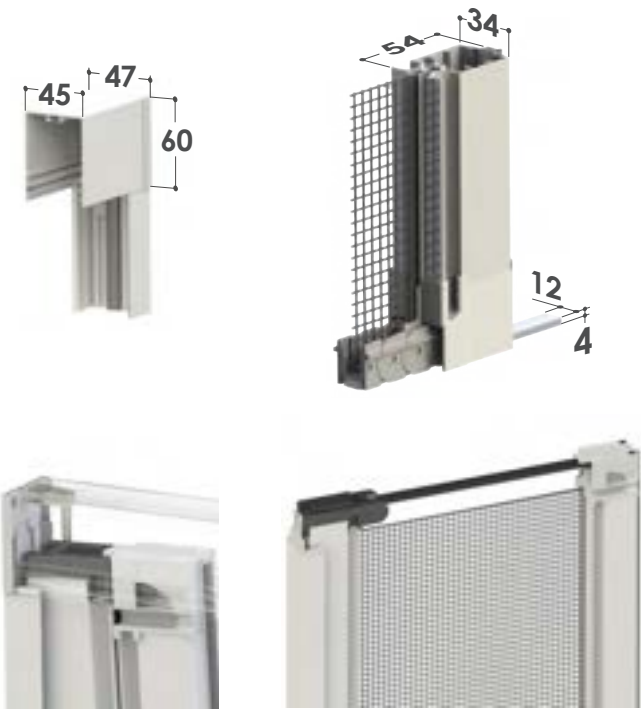
Conexión a bayoneta
