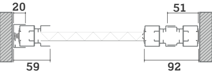
SECCIÓN HORIZONTAL 2 HOJAS SEGUIDAS
