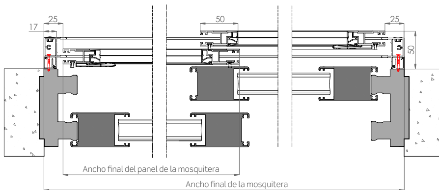
Sección horizontal
