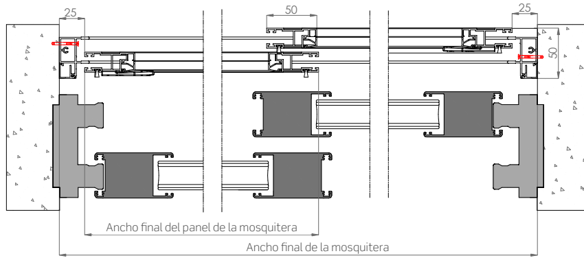
Sección horizontal
