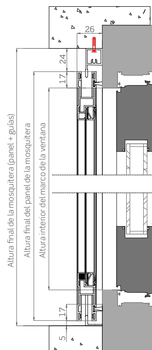
Sección vertical
