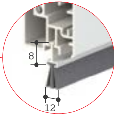
Barra con manija y perfil portacepillos telescópico (hasta 8 mm).
