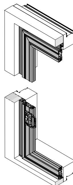
Sección vertical
