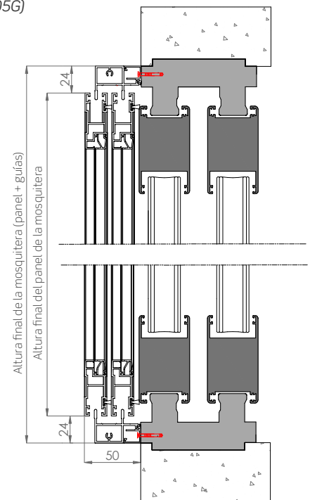
Sección vertical
