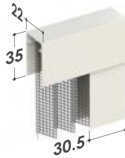
Sistema de drenaje del agua
