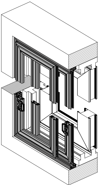
Sección vertical
