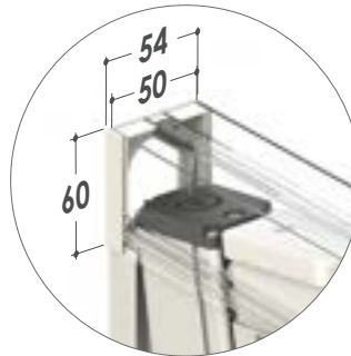
Conexión de bayoneta con guía ESTÁNDAR y de imán con guía MIDI
