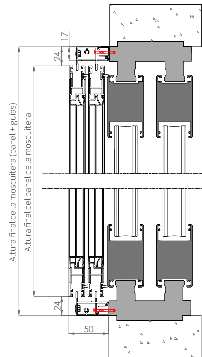
Sección vertical
