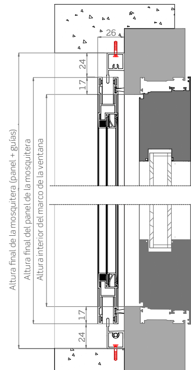
Sección vertical
