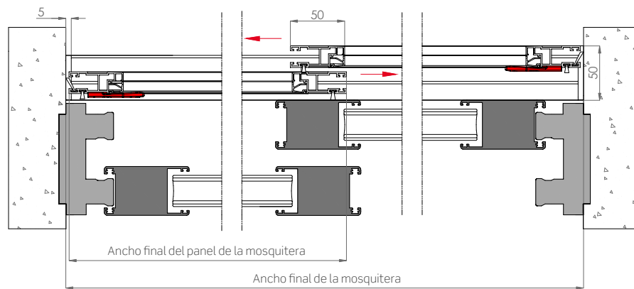
Sección horizontal
