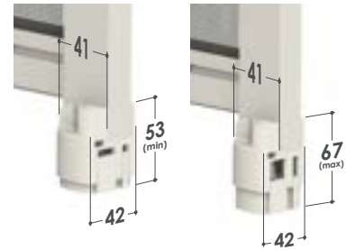
Pies de expansión de serie, apertura máxima
