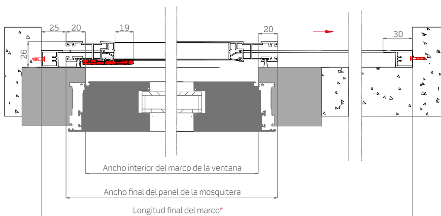
Sección horizontal
