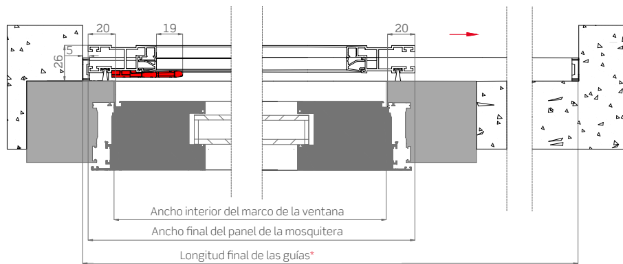
Sección horizontal
