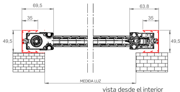
vista desde el interior
