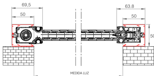
vista desde el interior
