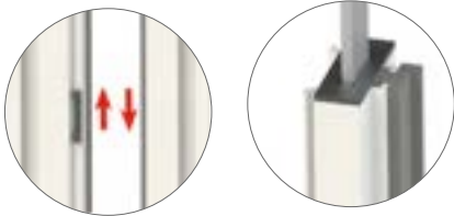
SISTEMA DE BLOQUEO CON PASADOR
