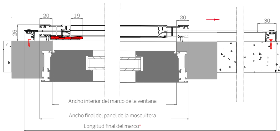
Sección horizontal
