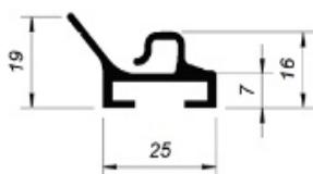
Terminal de Goma TR-125
