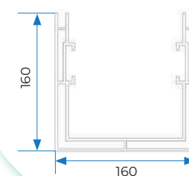
A2 PERFIL PILAR U
