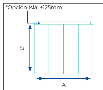
Estructura Seesky LUZ en configuración isla
