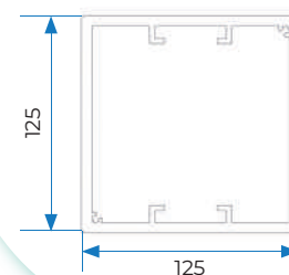
A2 PERFIL PILAR CERRADO
