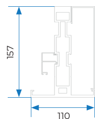
7 GUIA LATERAL PANEL FIJO
