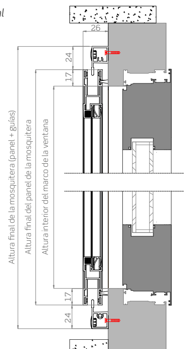
Sección vertical
