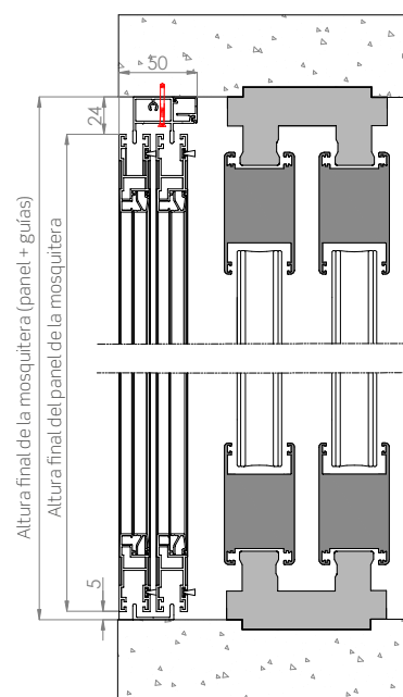
Sección vertical
