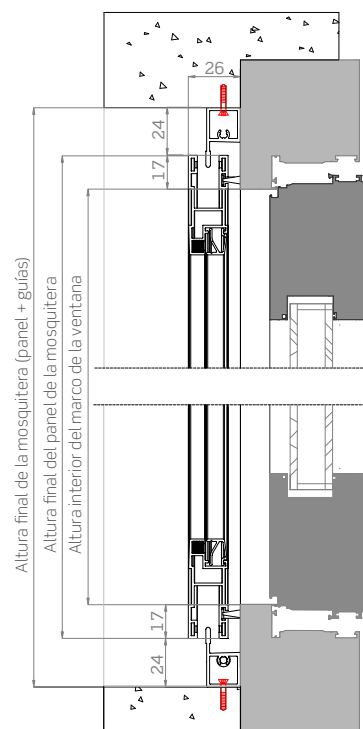
Sección vertical
