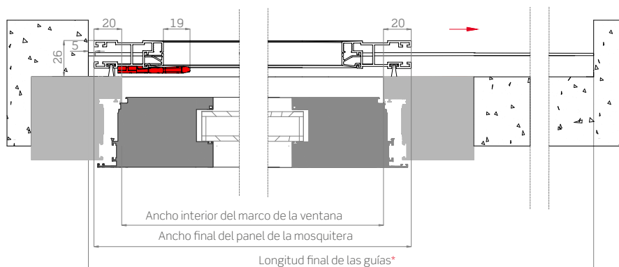
Sección horizontal
