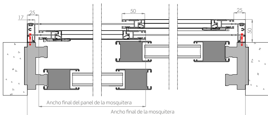
Sección horizontal
