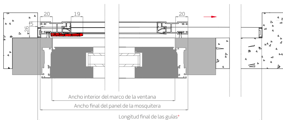
Sección horizontal
