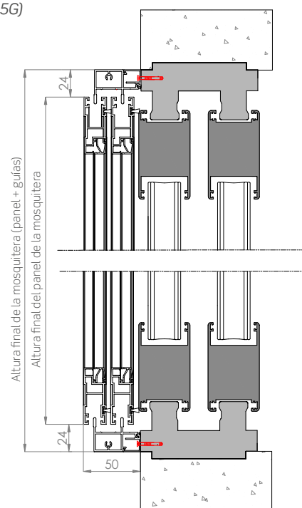
Sección vertical
