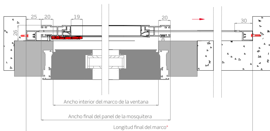
Sección horizontal
