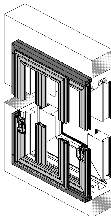
Sección vertical
