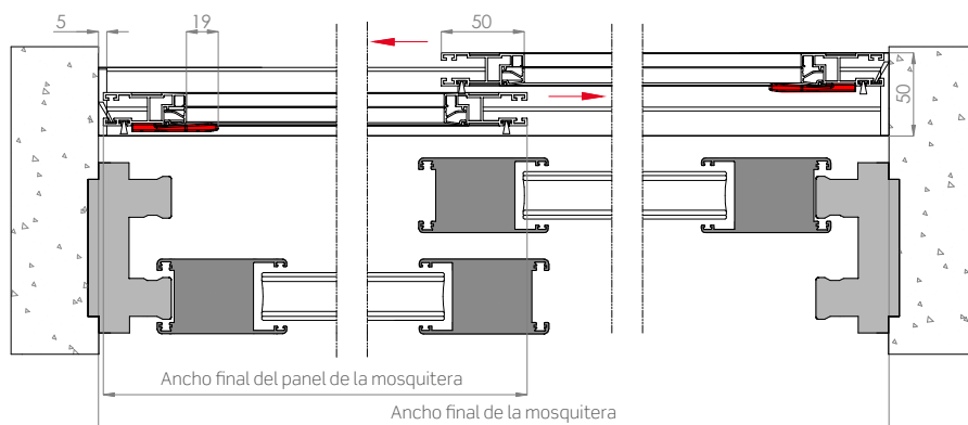
Sección horizontal
