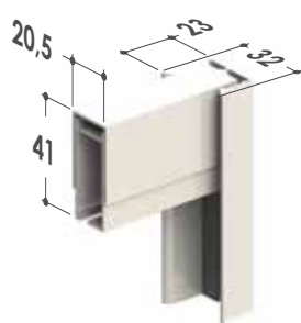
Guías telescópicas ajustables
