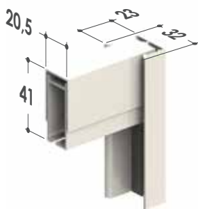
Guías telescópicas ajustables
