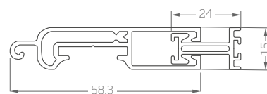
Terminal con perfil telescópico
