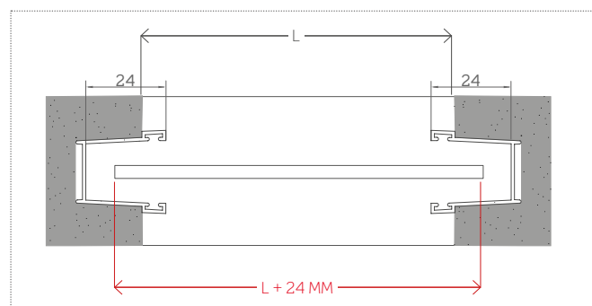
AT36015 - Instalación empotrada
