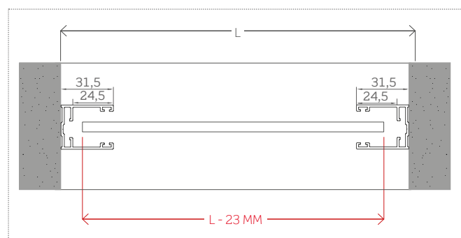
AT34006 - Instalación empotrada
