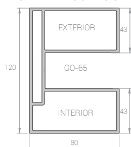
DOBLE ALOJA-GUÍAS
