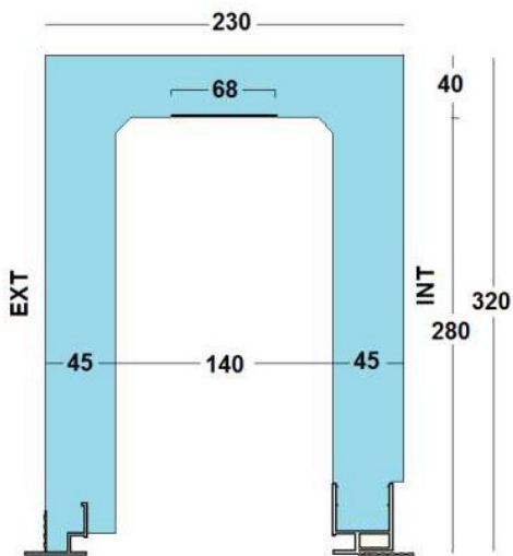
CAJAISLANT® SHADOW 230
