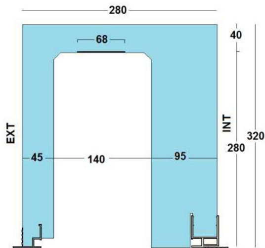
CAJAISLANT® SHADOW 280
